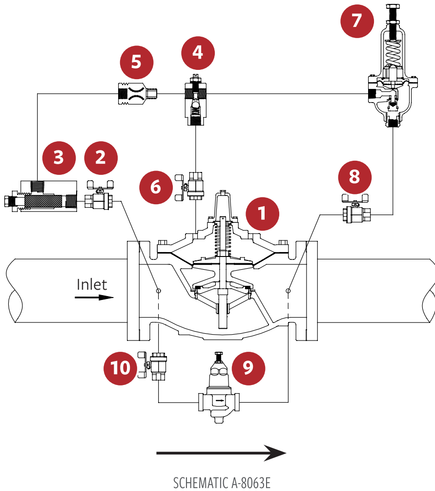
FIG. 2 Schematic A-8063E
